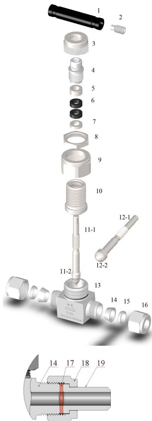
活接对焊型式 Union butt welding type
